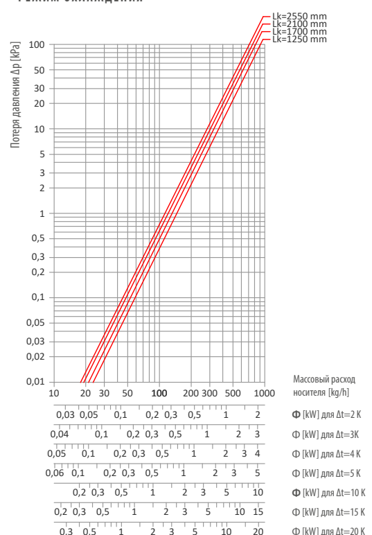
СVK4-18/35/Lk-II РЕЖИМ ОХЛАЖДЕНИЯ
