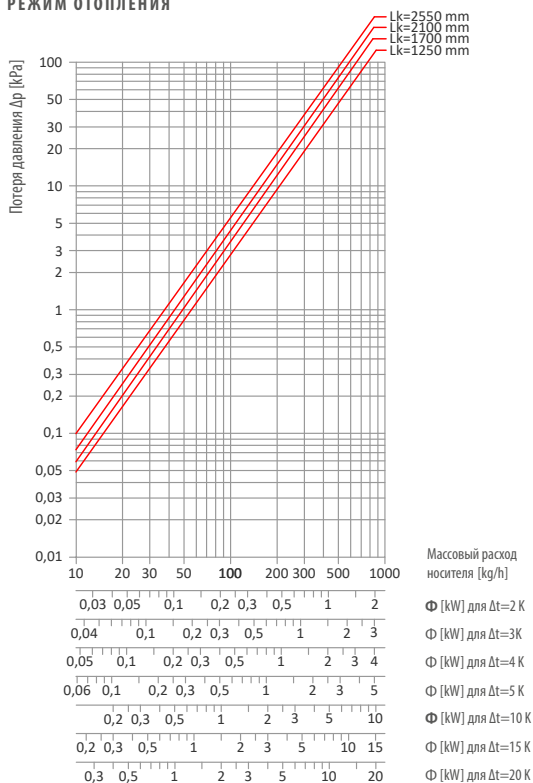
CVK4-14/35/Lk-II РЕЖИМ ОТОПЛЕНИЯ
