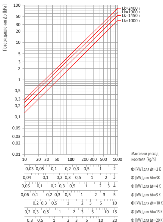
СVK4-18/35/Lk-1 РЕЖИМ ОТОПЛЕНИЯ
