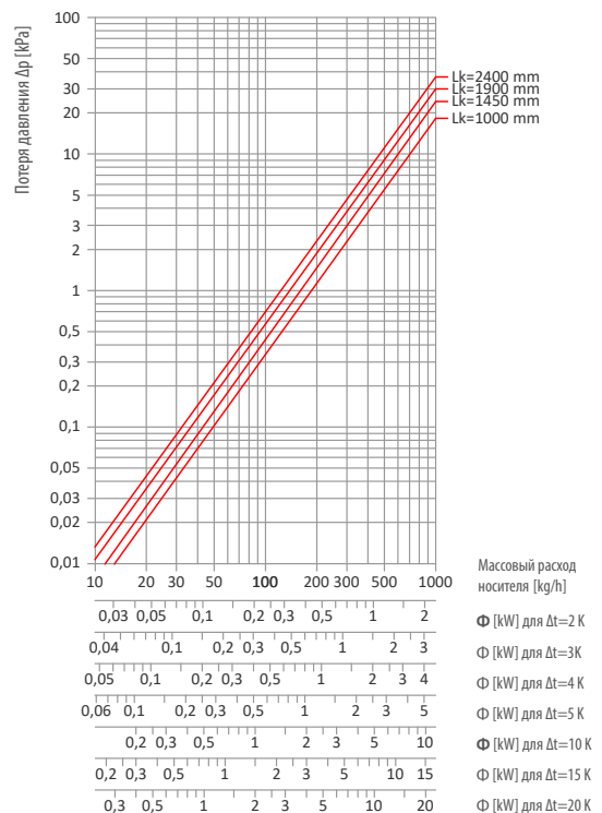
SVK4-14/35/Lk-I РЕЖИМ ОХЛАЖДЕНИЯ
