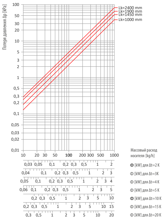
SVK4-14/35/Lk-I РЕЖИМ ОТОПЛЕНИЯ
