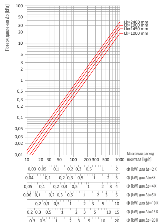
СVK4-18/35/Lk-1 РЕЖИМ ОХЛАЖДЕНИЯ
