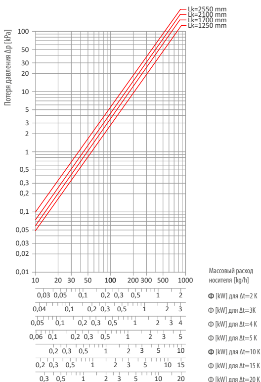
СVK4-18/35/Lk-II РЕЖИМ ОТОПЛЕНИЯ
